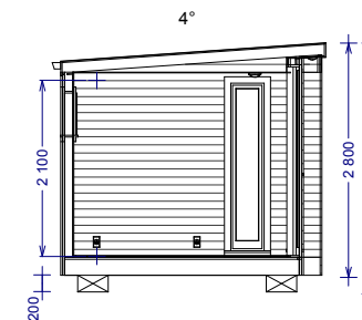
SEKTION
