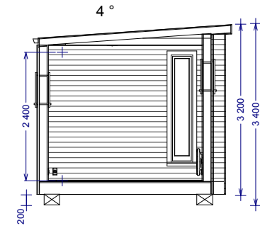
SEKTION
