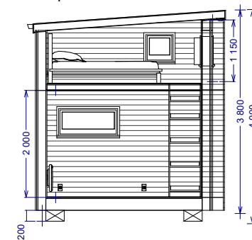
Sektion, a-a
