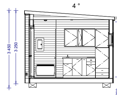
SEKTION
