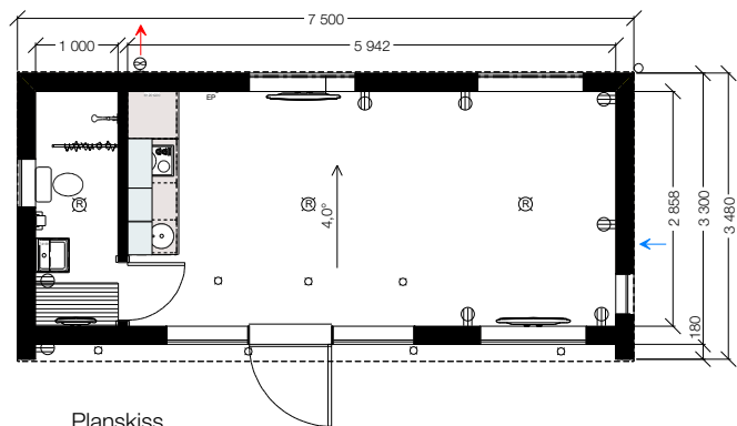
Planskiss
