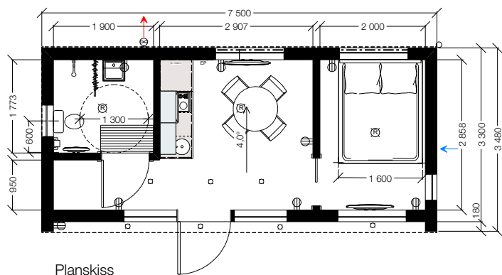
Planskiss
