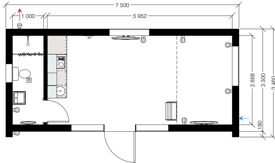
E25 Loft ST1 Entréplan
